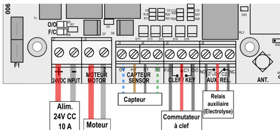
Schéma de câblage coffret AN2010
